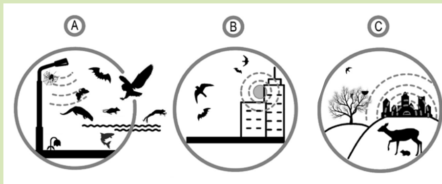
Obrázek 3: Příklady účinků umělého nočního osvětlení na organismy
