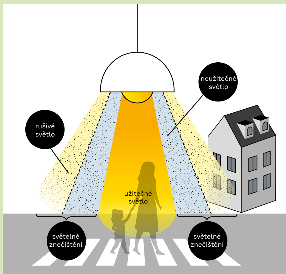
Obrázek 2: Schematické znázornění světelného znečištění
